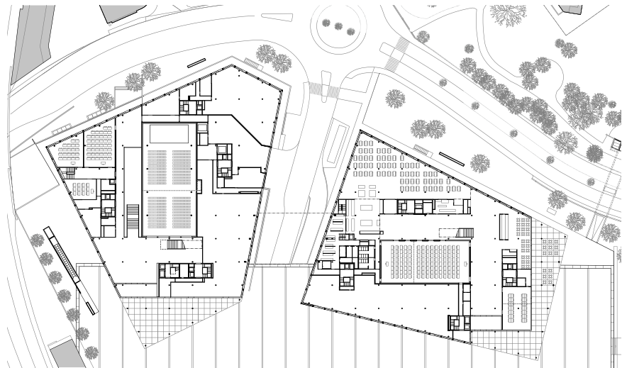
Erdgeschoss
