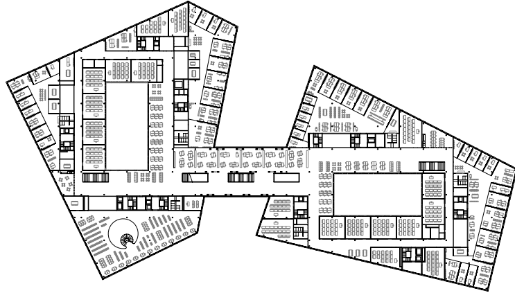
3. Obergeschoss
