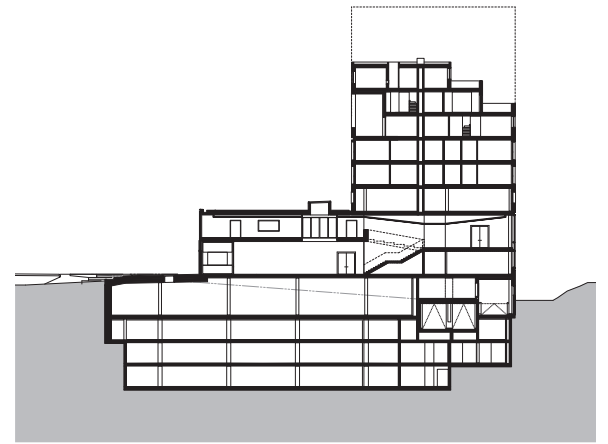
Querschnitt
