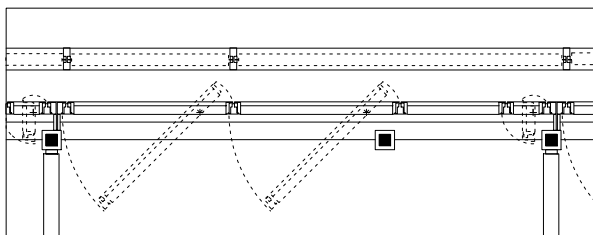
NOUVELLE FAÇADE AVEC DES OU- VERTURES À BATTANTS POUR UNE UTILISATION OPTIMALE DE LA LU- MIÈRE DU JOUR ET DES CLAPETS POUR LA VENTILATION NOCTURNE PASSIVE. STORES EXTÉRIEURS
