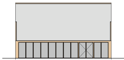
Façade Est
